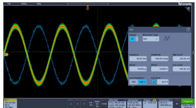
Гибкая настройка генератора сигналов произвольной формы. В данном случае к синусоидальному сигналу добавлено 20 % шума.
