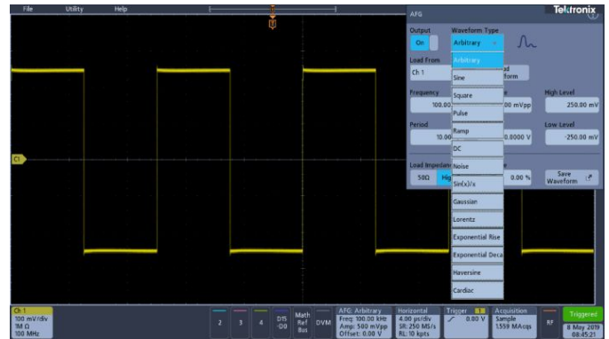
Выбор типа сигнала во встроенном генераторе сигналов произвольной формы и стандартных функций.
