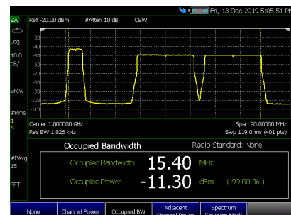
Измерение занимаемой полосы частот для сигнала LTE-A
